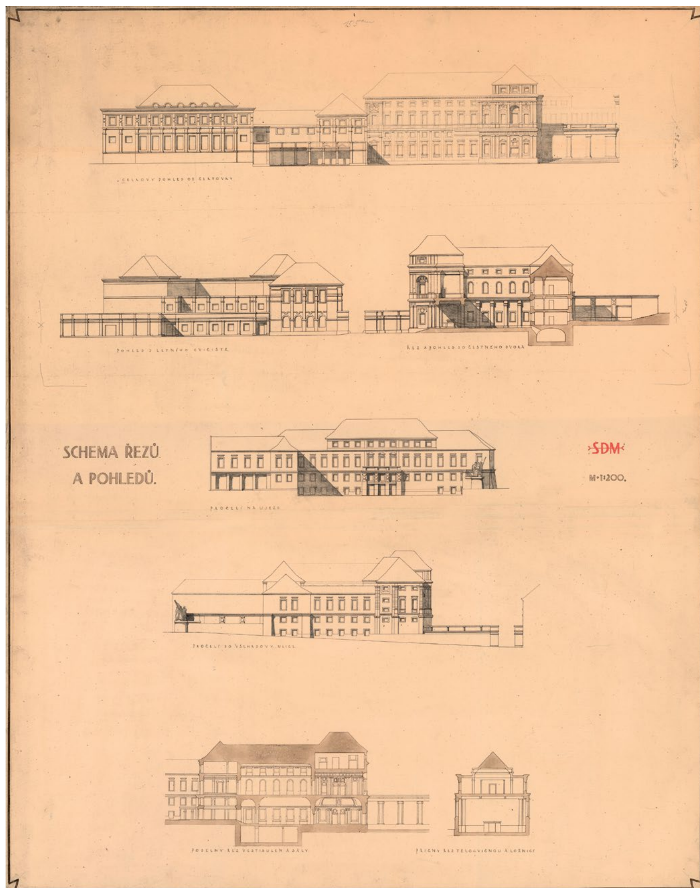
Soutěžní návrh na přestavbu Tyršova domu s heslem „SDM“
